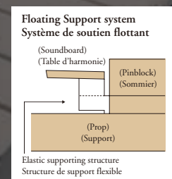
Structure de la console de la table d'harmonie d'un piano droit
