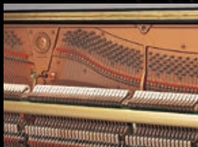
High-quality agraffes and CFX spec hammers Agrafes haut de gamme et marteaux aux caractéristiques CFX
